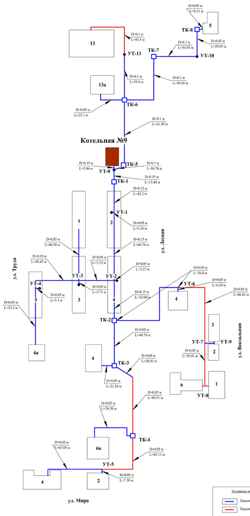
Рис. 2 - Схема тепловых сетей Котельной №9 ст. Железнодорожная станция Алнаши
